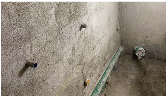
Mit FM 388 Light fertig verputzte Wand vor dem Aufbringen der Gewebespatchtelung mit codeX UX 410 und einem codeX Dünnbettmörtel
