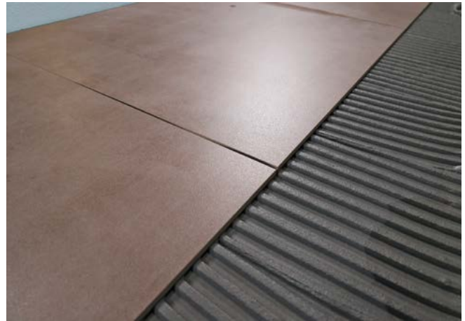
Fliesen verlegt mit codex Power RX 11 Outdoor bereits nach 6 Stunden verfügar
