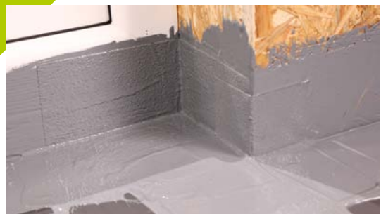
Die zweite Schicht erfolgt direkt im Anschluss Frisch-in-Frisch
