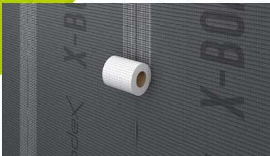
Bauplattenstöße mit codex Stoßband fixieren. Im Nassbereich durch das codex Dichtband ersetzen
