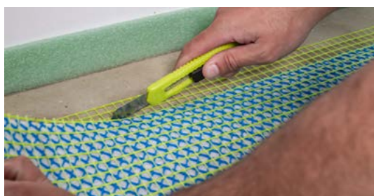
1. Vor Verlegung der ersten Reihe den Überstand mit Messer oder Schere abschneiden
